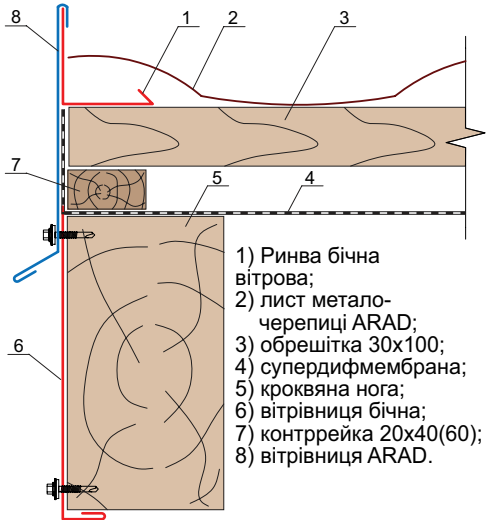
Рис. 2.1. Вітровий вузол
